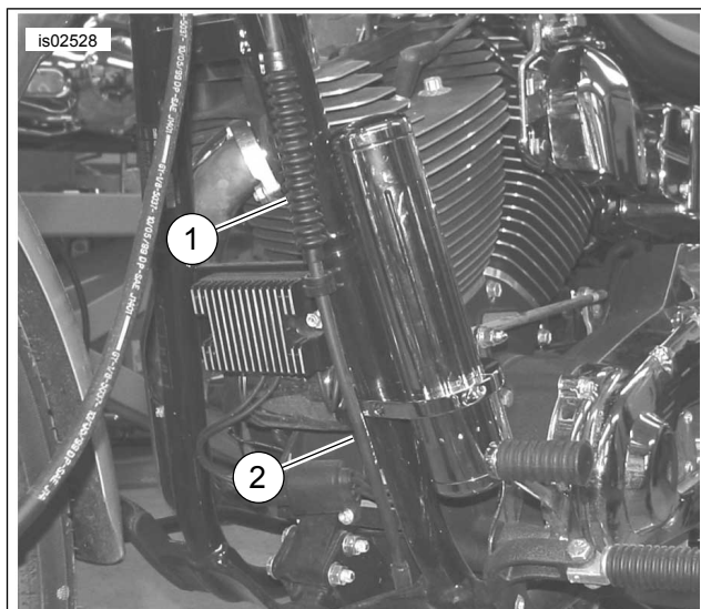
1. Cable adjuster 2. Clutch cable
